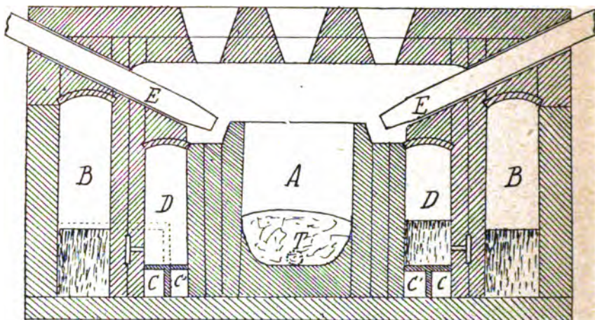
Fig. 159. — Four mixte système Minet.
